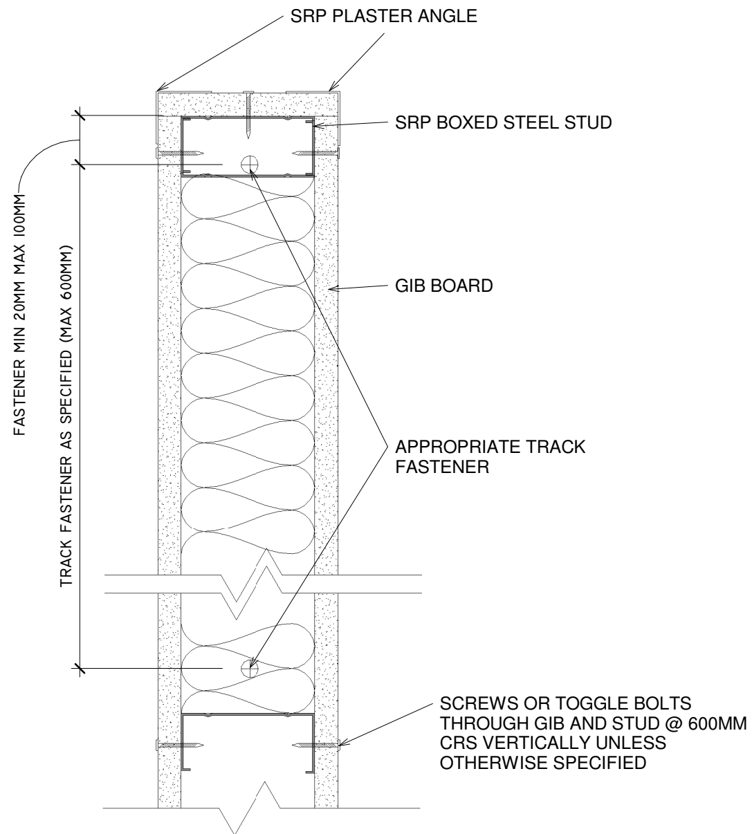
SRP BOXED STUD OPEN END
